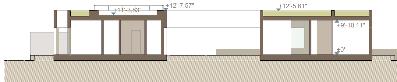
S-02 SECTION
